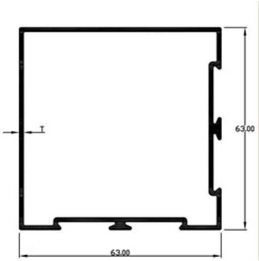
DOOR SECTION
