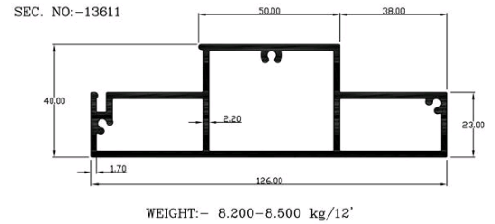
DOOR SECTION
