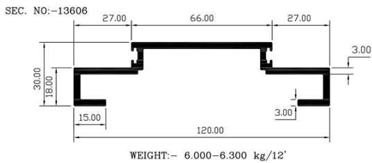
DOOR SECTION
