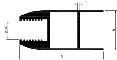
FISHTYPE DOOR BOTTOM
